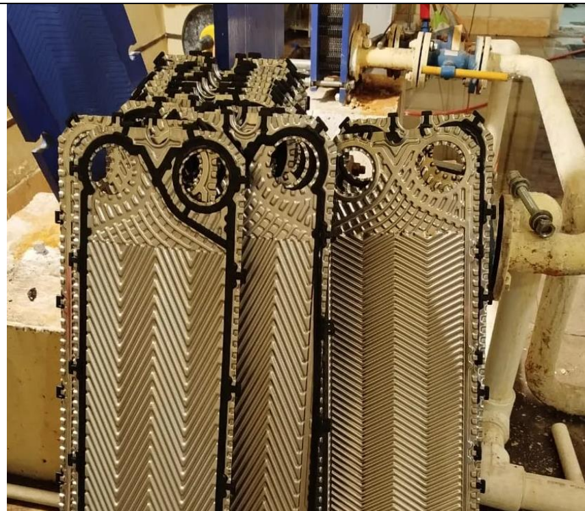
Промывка теплообменника
