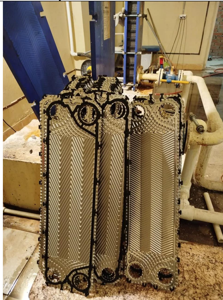
Промывка теплообменника.
