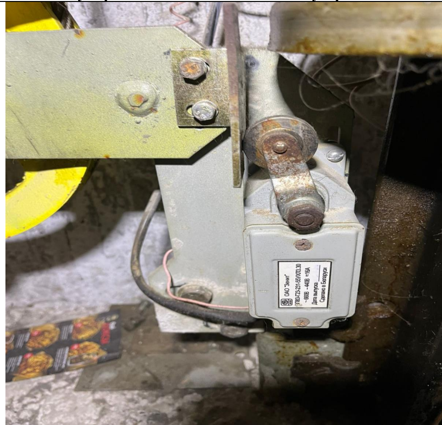
Регулировка концевика натяжного устройства
