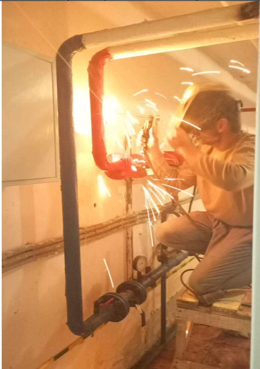
Вваривание резьбы на тепломагистраль
